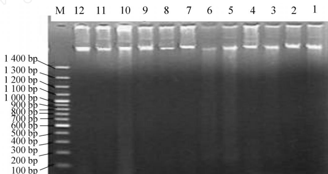
图 2 雄蜂 DNA 电泳图
