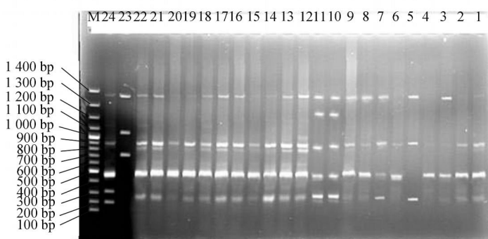
图 3 引物 A1 扩增电泳图 (无螨雄蜂)
